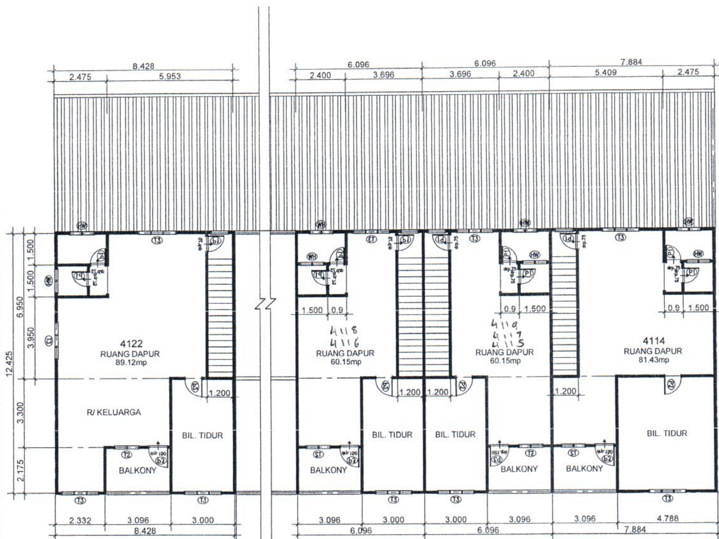
Pelan Lantai Tingkat Atas PERKEDAIAN PASIR AKAR, BESUT
